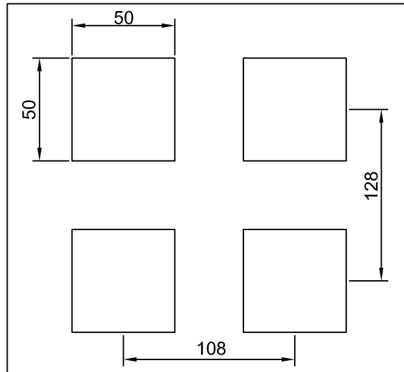
Fundamentplan Rondo
